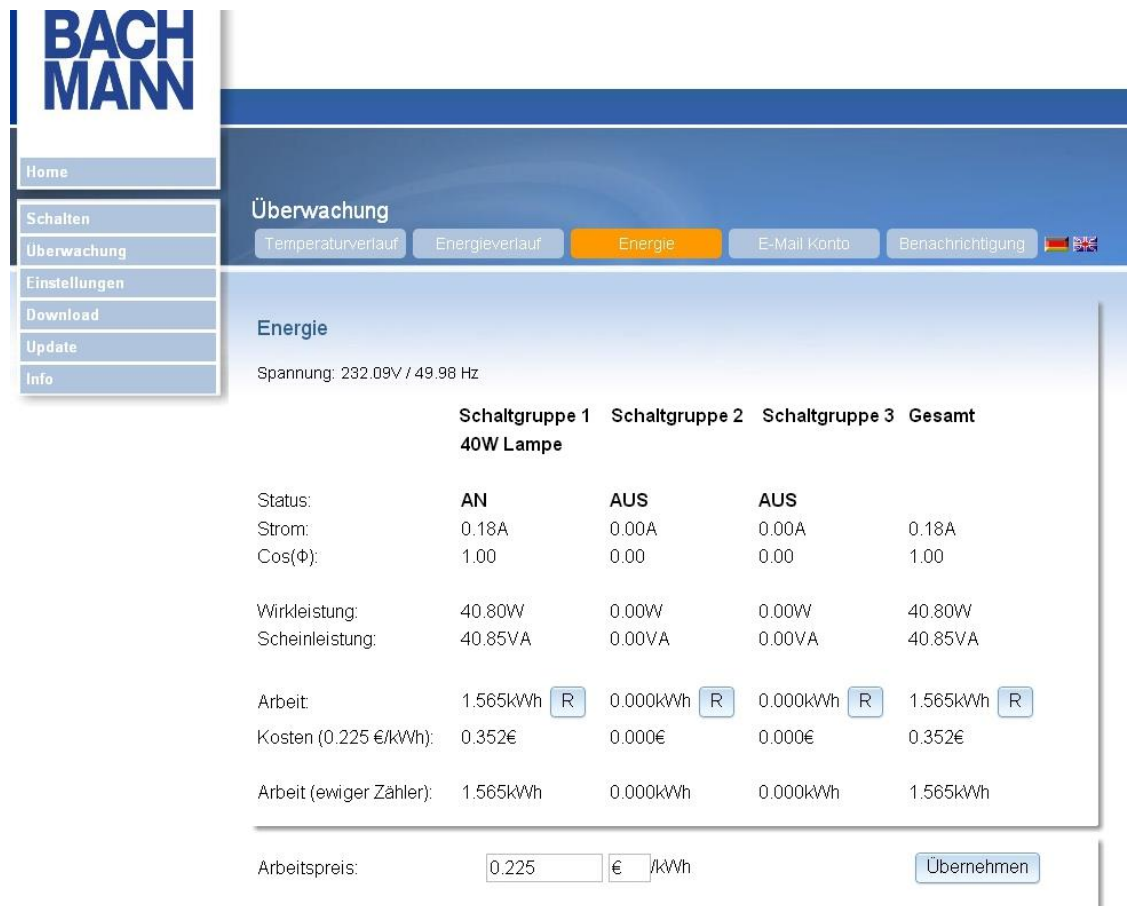
Abbildung 20: Leistungsaufnahme
