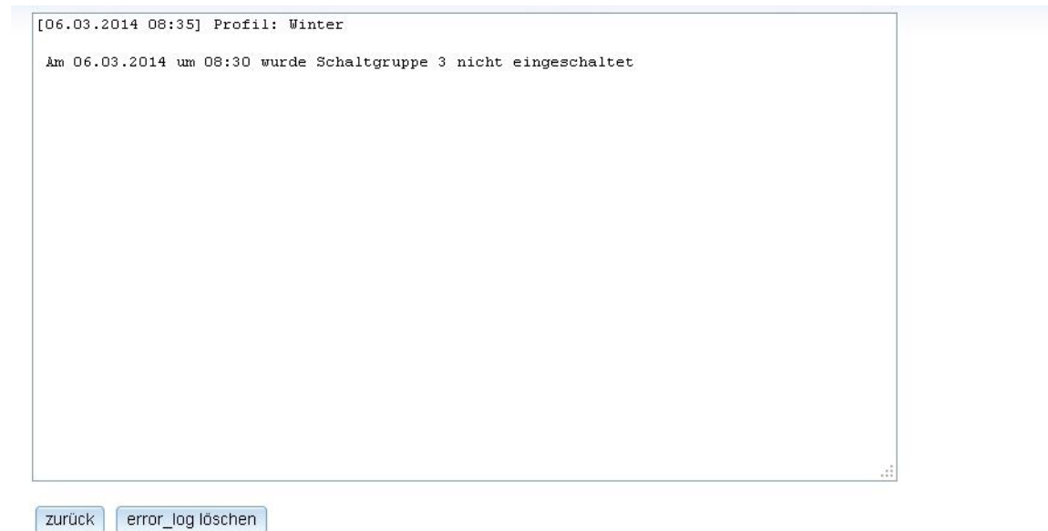
Abbildung 15: error_log anzeigen
