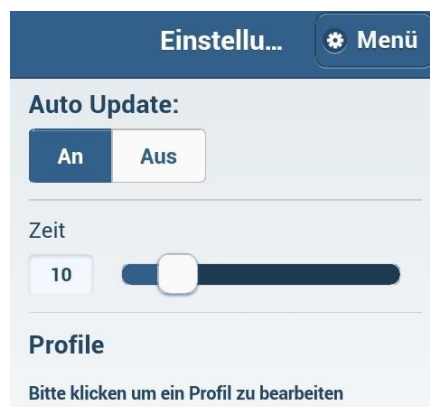
Abbildung 1: Einstellbildschirm
