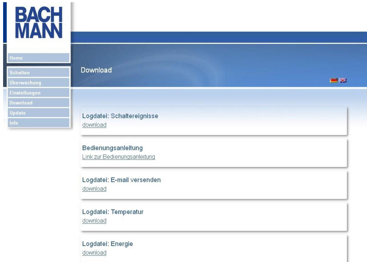
Abbildung 23: Download Logdateien
